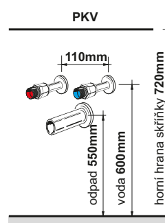
MONTÁŽNÍ VÝŠKA
