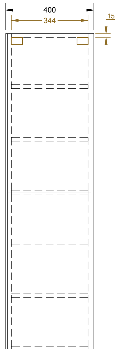
PŘEDNÍ POHLED
