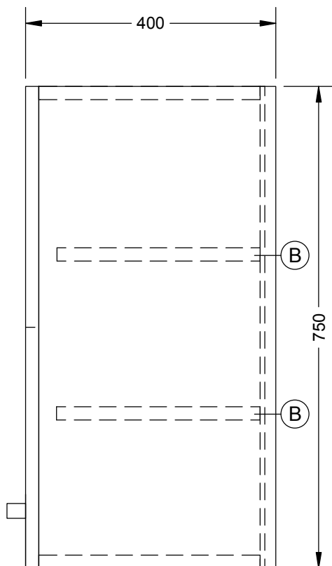
BOČNÍ POHLED
