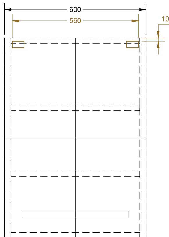
PŘEDNÍ POHLED
