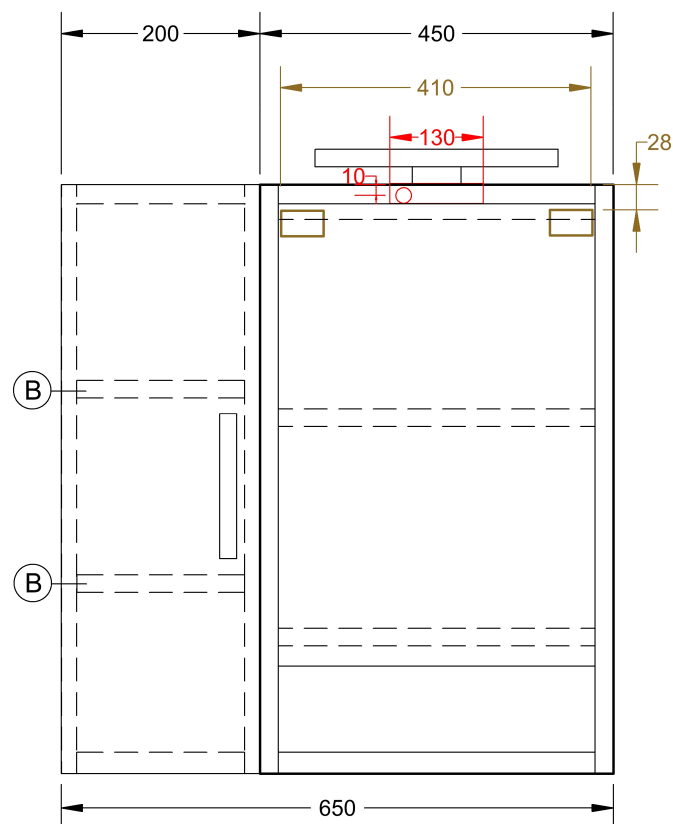
PŘEDNÍ POHLED
