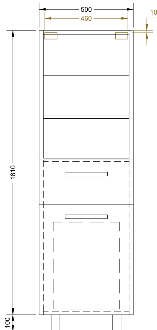
PŘEDNÍ POHLED
