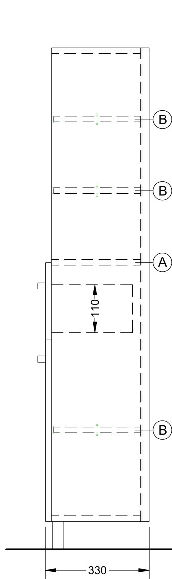
BOČNÍ POHLED
