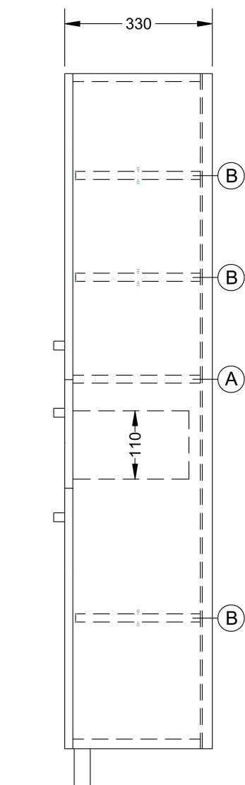
BOČNÍ POHLED
