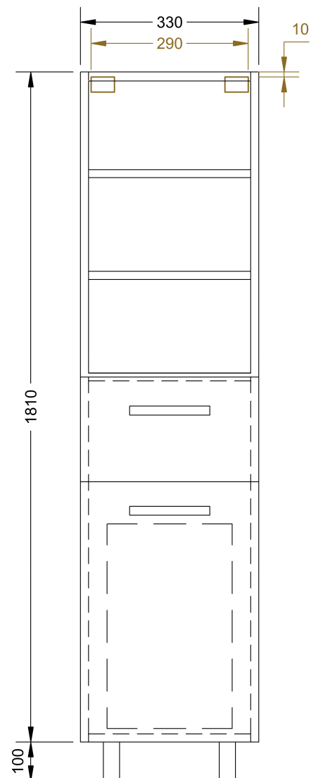
PŘEDNÍ POHLED
