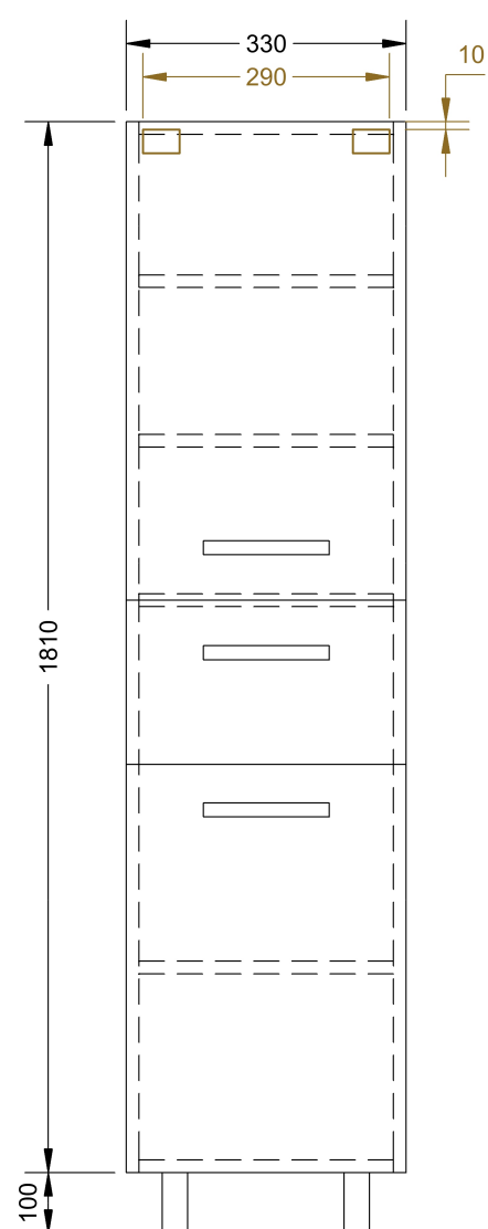
PŘEDNÍ POHLED
