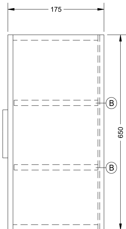
BOČNÍ POHLED
