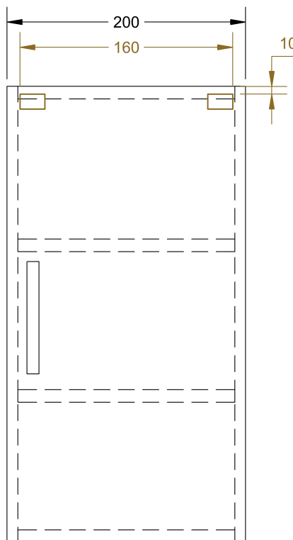
PŘEDNÍ POHLED
