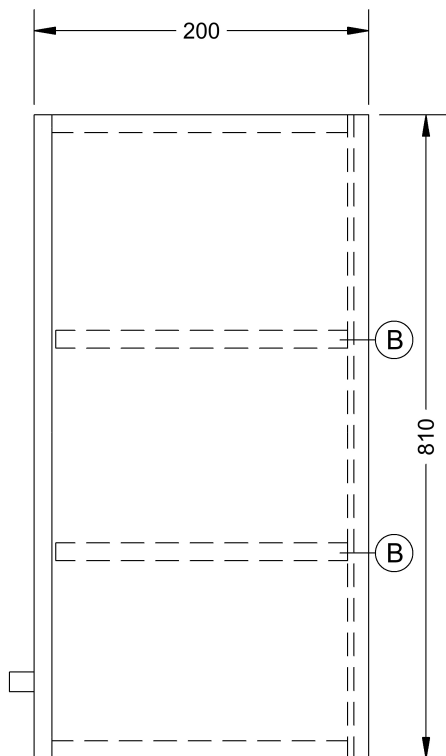
BOČNÍ POHLED
