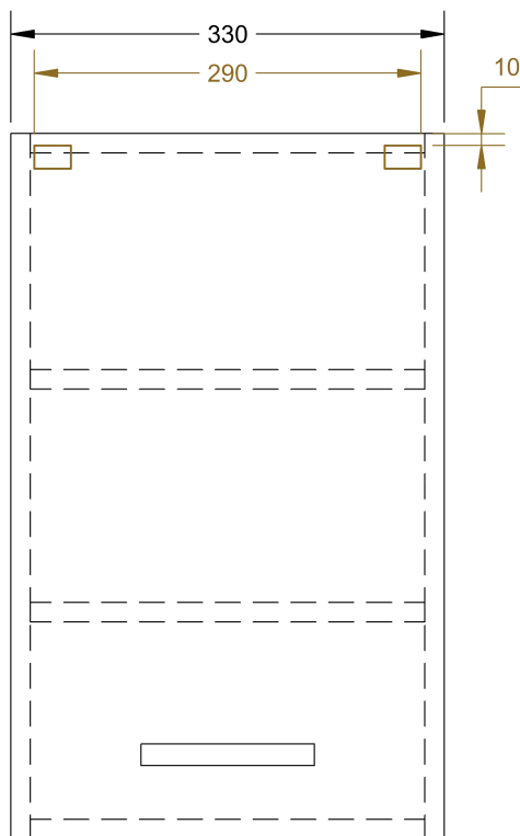
PŘEDNÍ POHLED
