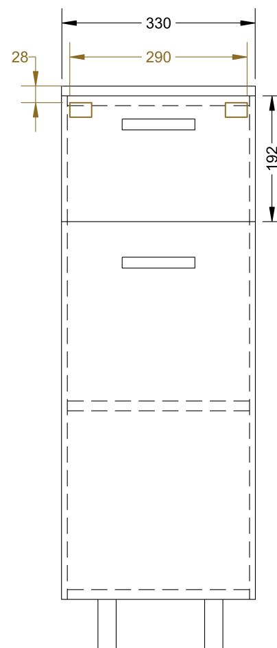
PŘEDNÍ POHLED
