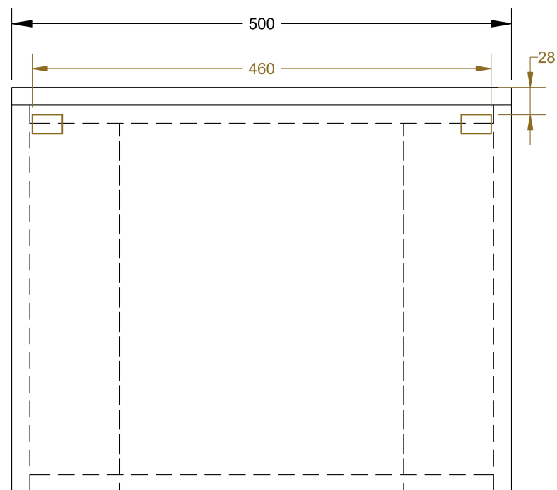
PŘEDNÍ POHLED
