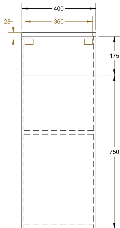
PŘEDNÍ POHLED
