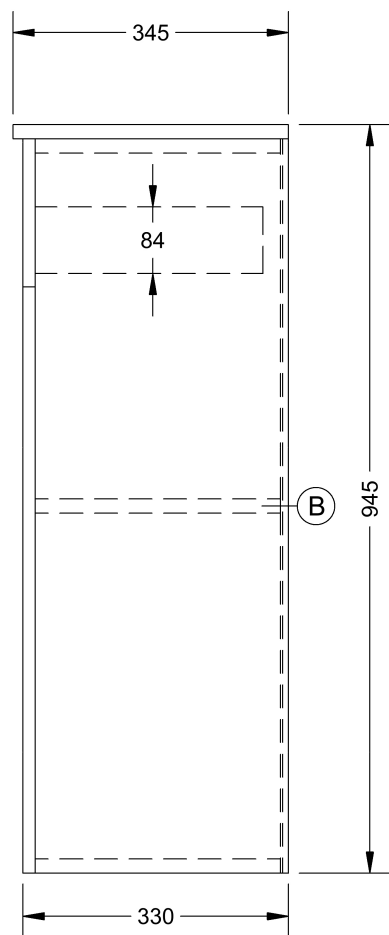
BOČNÍ POHLED
