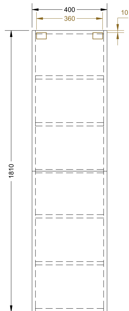
PŘEDNÍ POHLED
