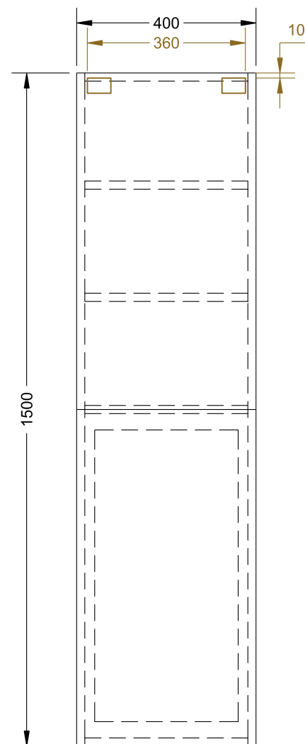
PŘEDNÍ POHLED
