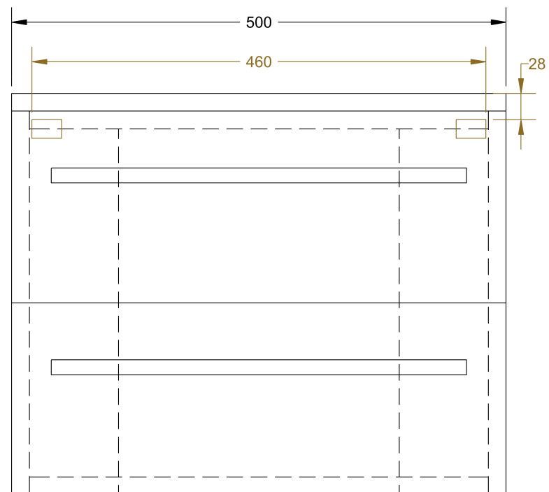
PŘEDNÍ POHLED
