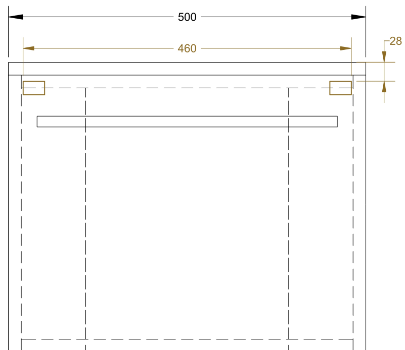
PŘEDNÍ POHLED
