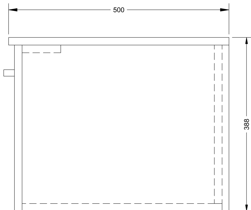
BOČNÍ POHLED
