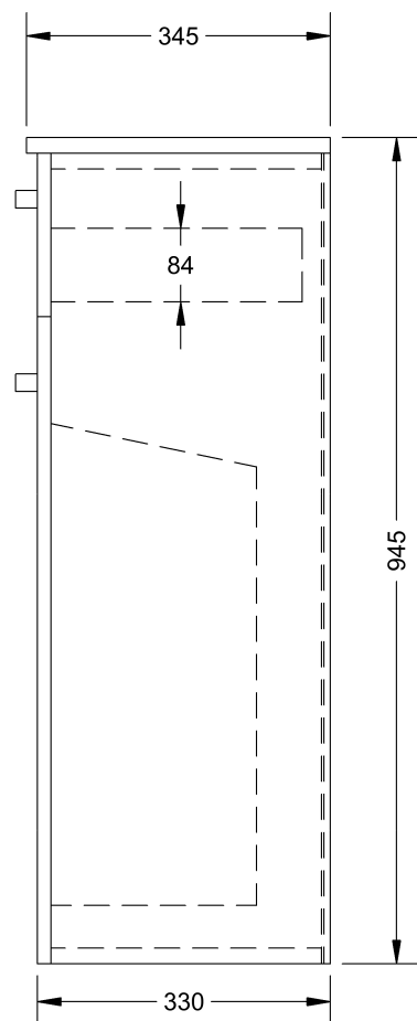
BOČNÍ POHLED
