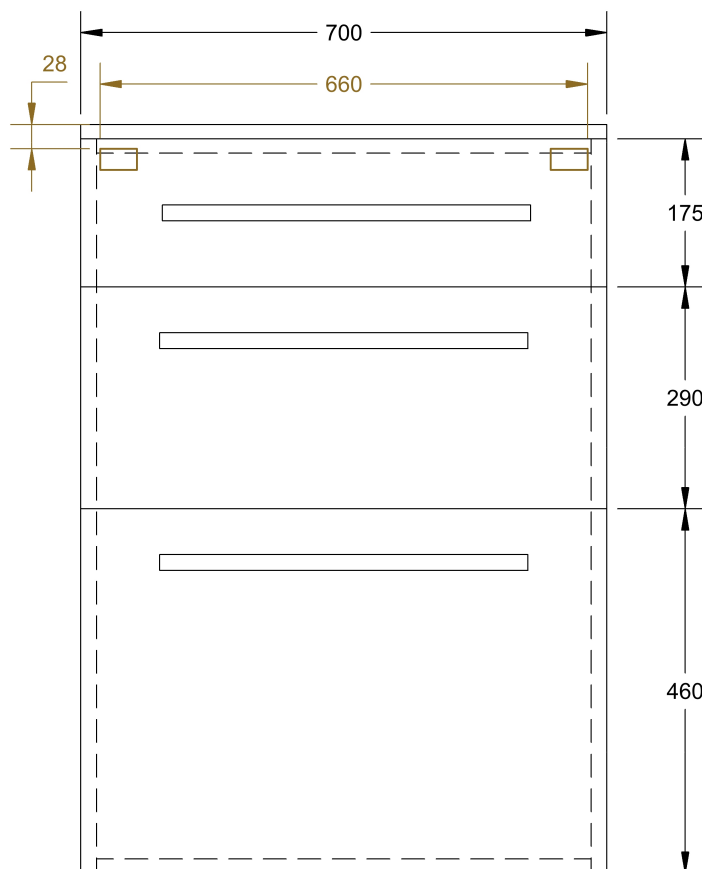
PŘEDNÍ POHLED
