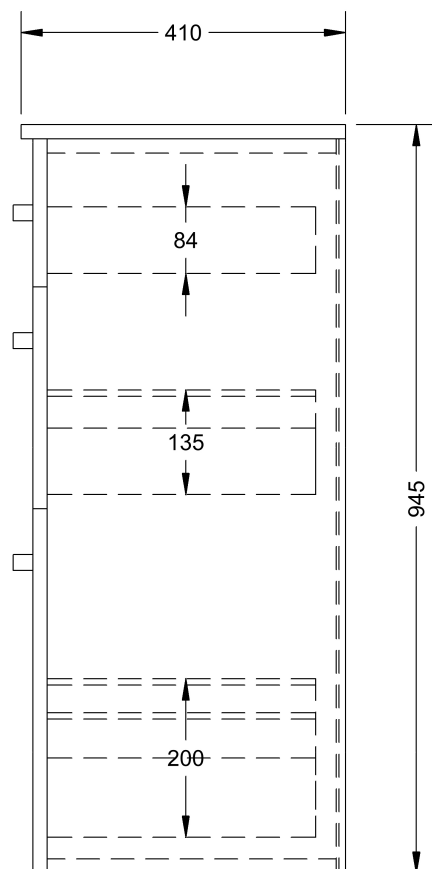
BOČNÍ POHLED
