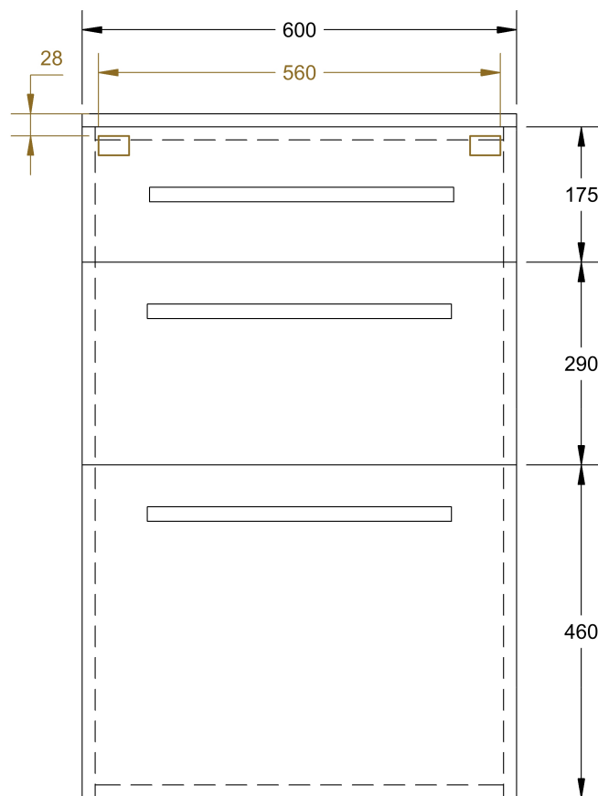
PŘEDNÍ POHLED
