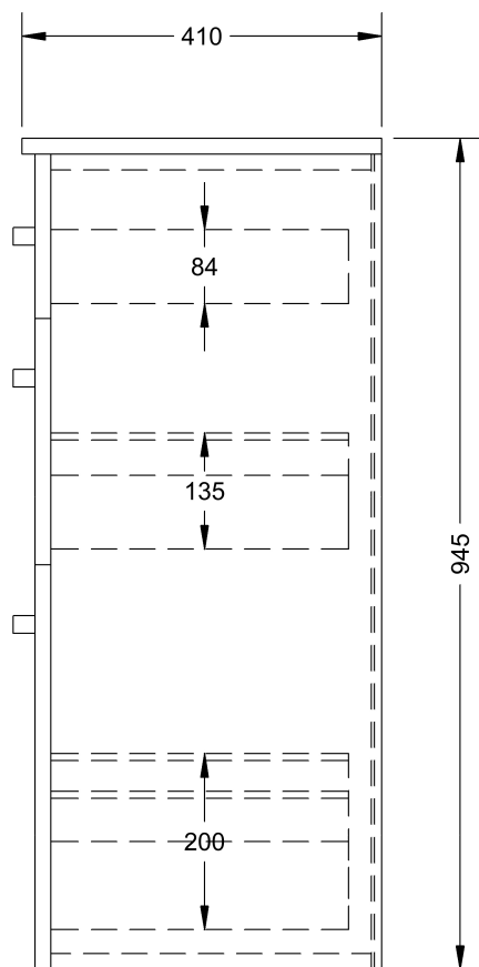
BOČNÍ POHLED
