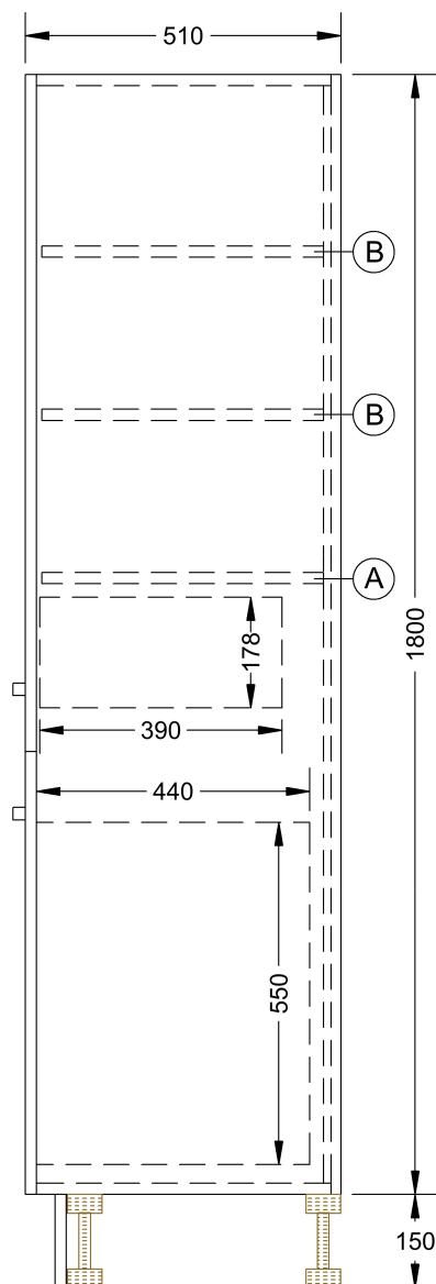
BOČNÍ POHLED
