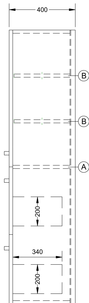
BOČNÍ POHLED
