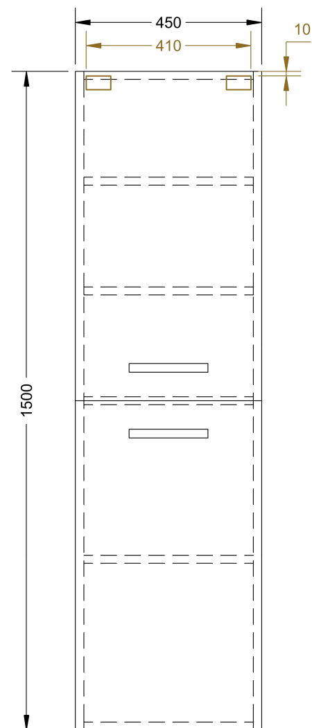
PŘEDNÍ POHLED
