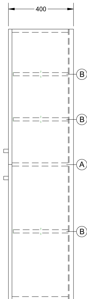
BOČNÍ POHLED
