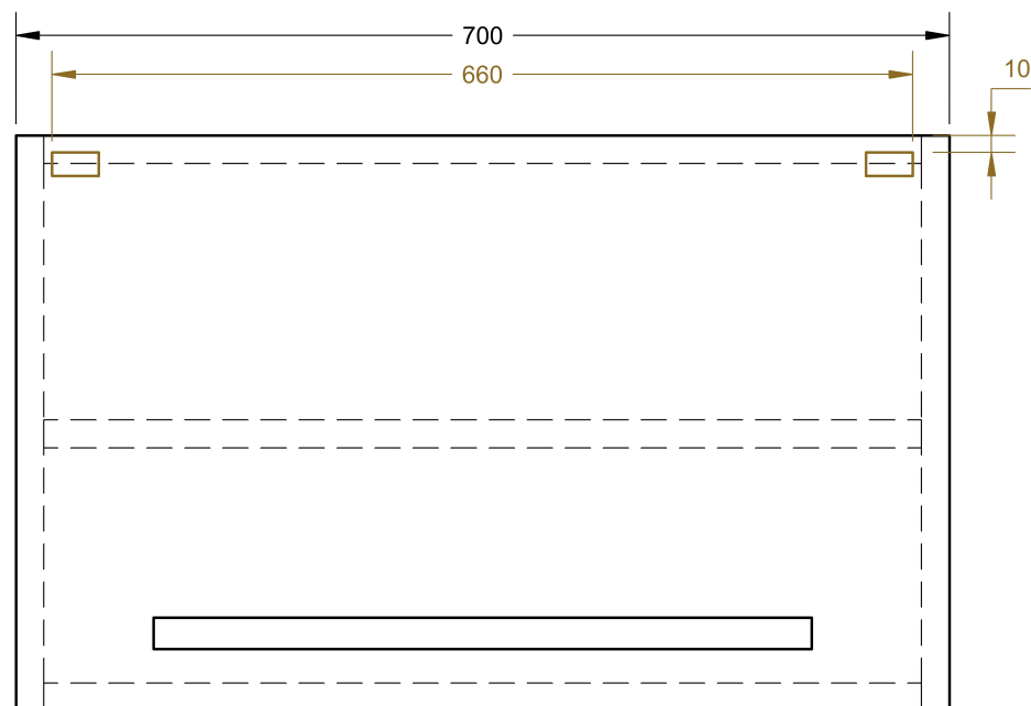
PŘEDNÍ POHLED
