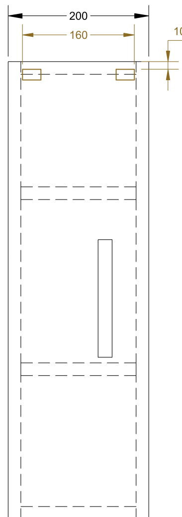
PŘEDNÍ POHLED
