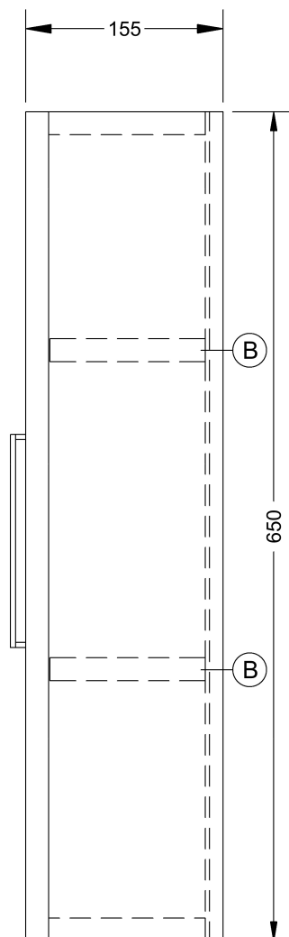
BOČNÍ POHLED
