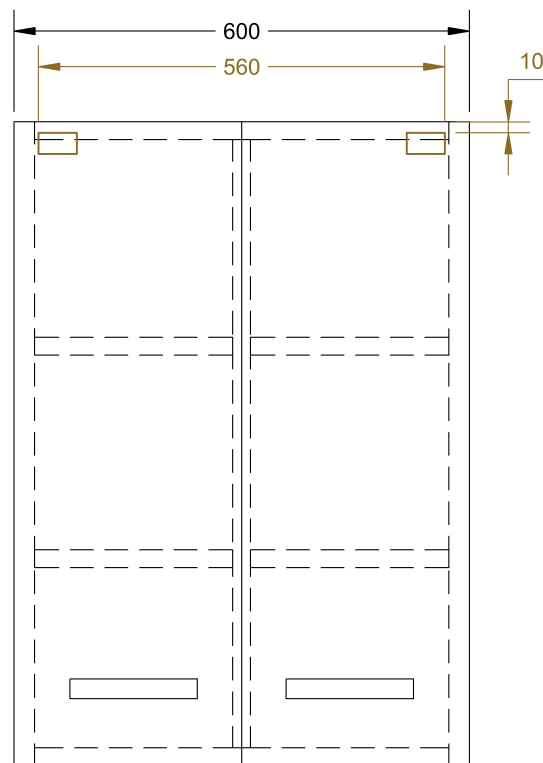
PŘEDNÍ POHLED
