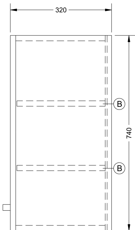
BOČNÍ POHLED
