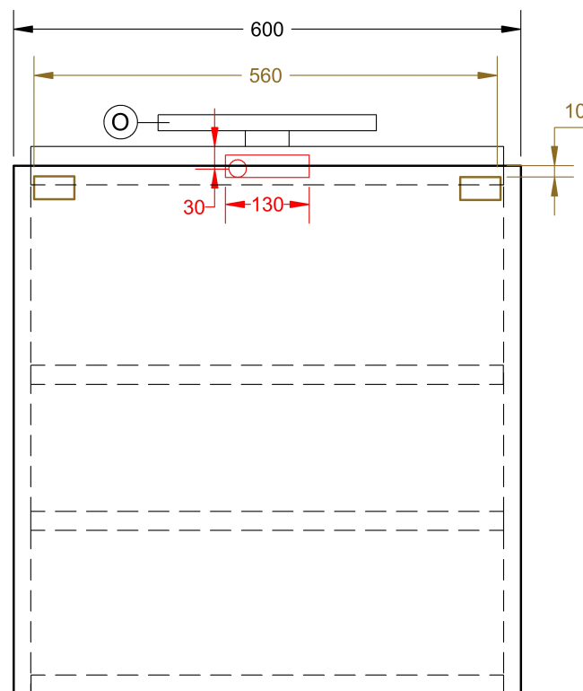
PŘEDNÍ POHLED
