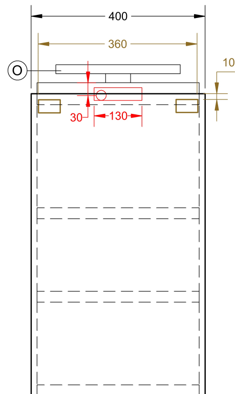
PŘEDNÍ POHLED
