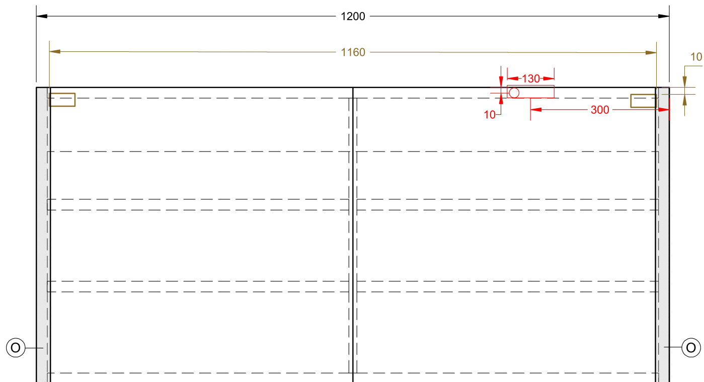
PŘEDNÍ POHLED
