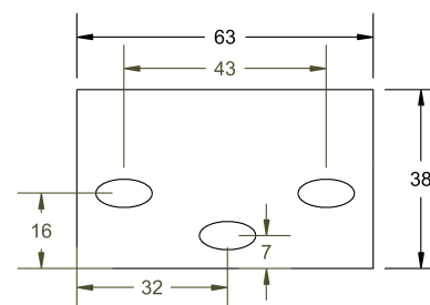
Detail profilu:
