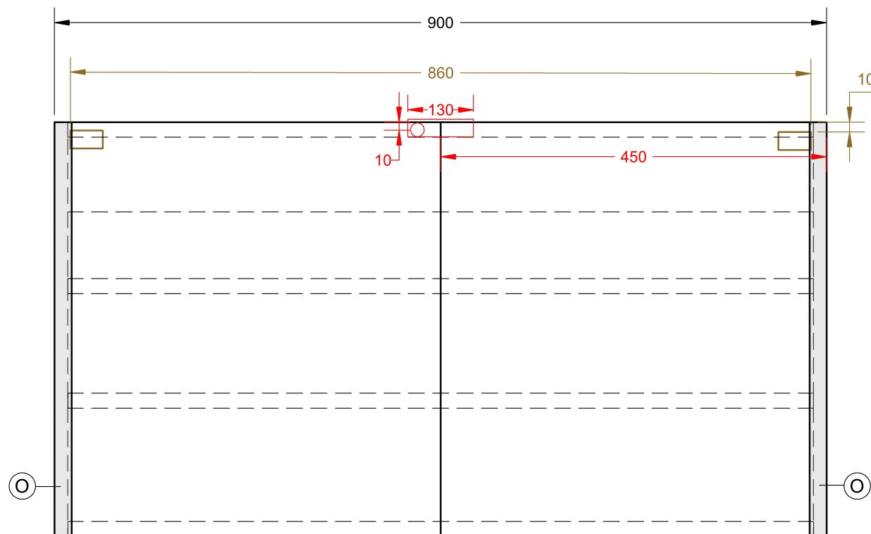
PŘEDNÍ POHLED
