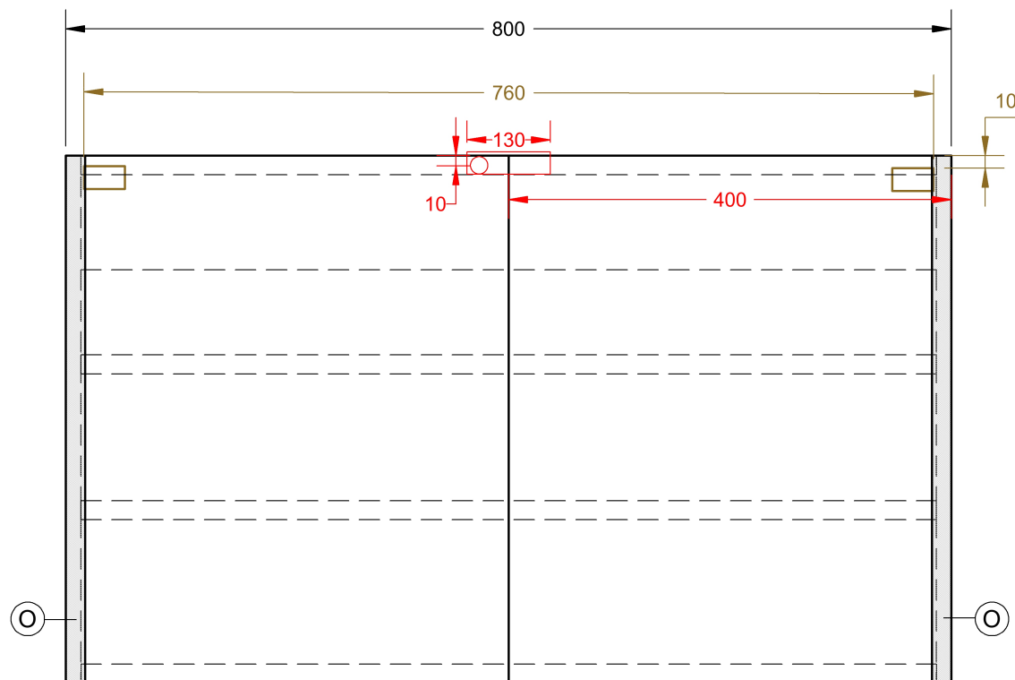
PŘEDNÍ POHLED
