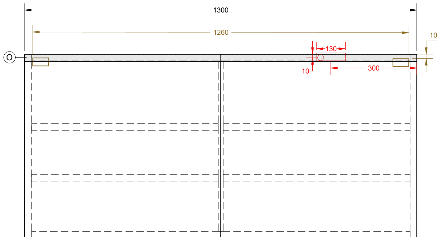
PŘEDNÍ POHLED
