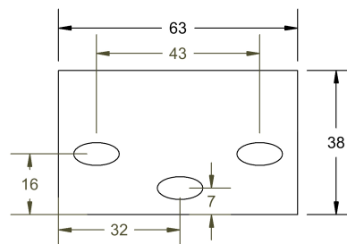
Detail profilu:
