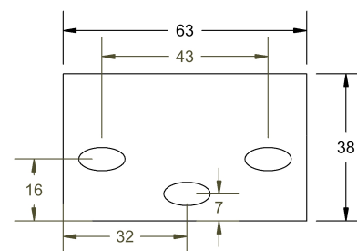
Detail profilu:
