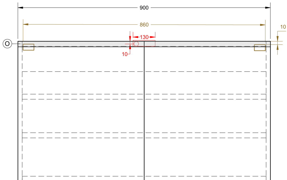
PŘEDNÍ POHLED
