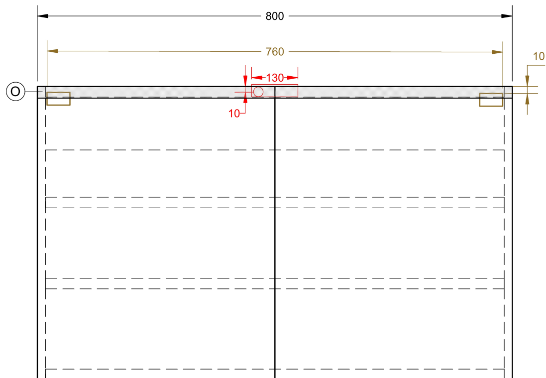
PŘEDNÍ POHLED
