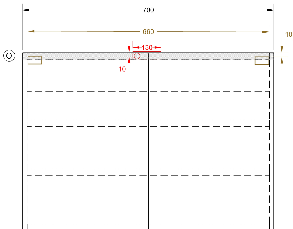
PŘEDNÍ POHLED
