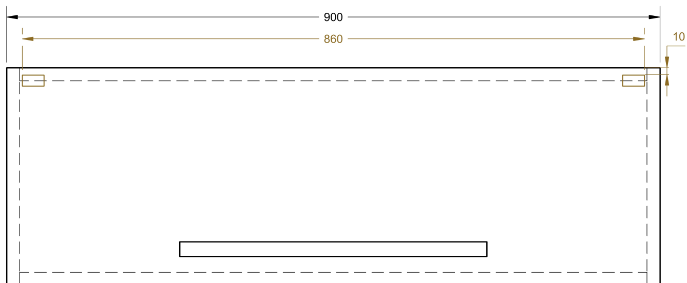
PŘEDNÍ POHLED
