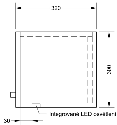
BOČNÍ POHLED
