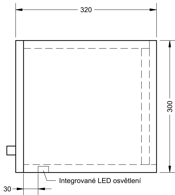
BOČNÍ POHLED
