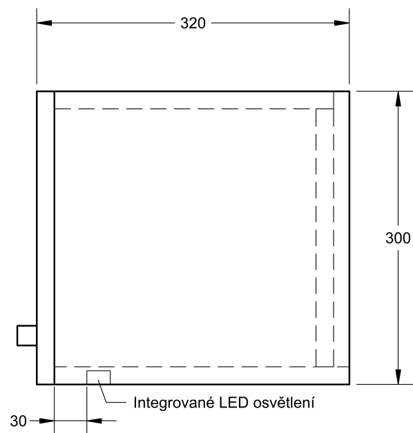
BOČNÍ POHLED
