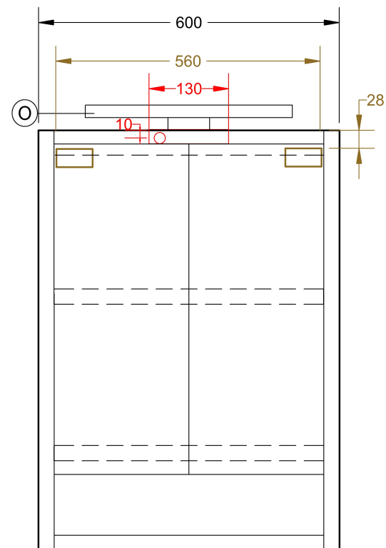
PŘEDNÍ POHLED
