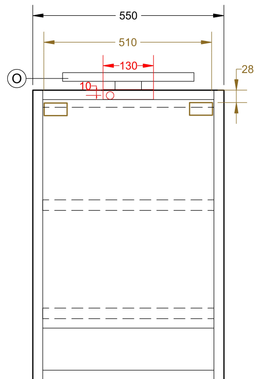
PŘEDNÍ POHLED
