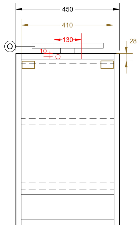
PŘEDNÍ POHLED
