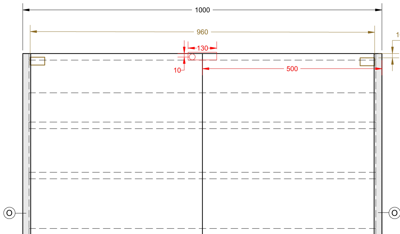
PŘEDNÍ POHLED
