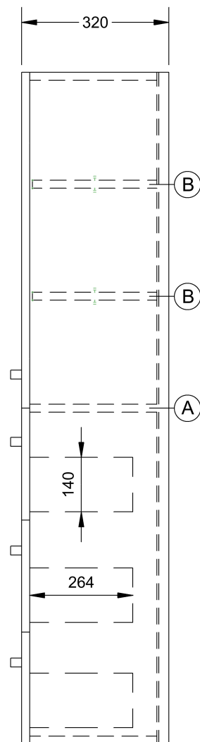
BOČNÍ POHLED
