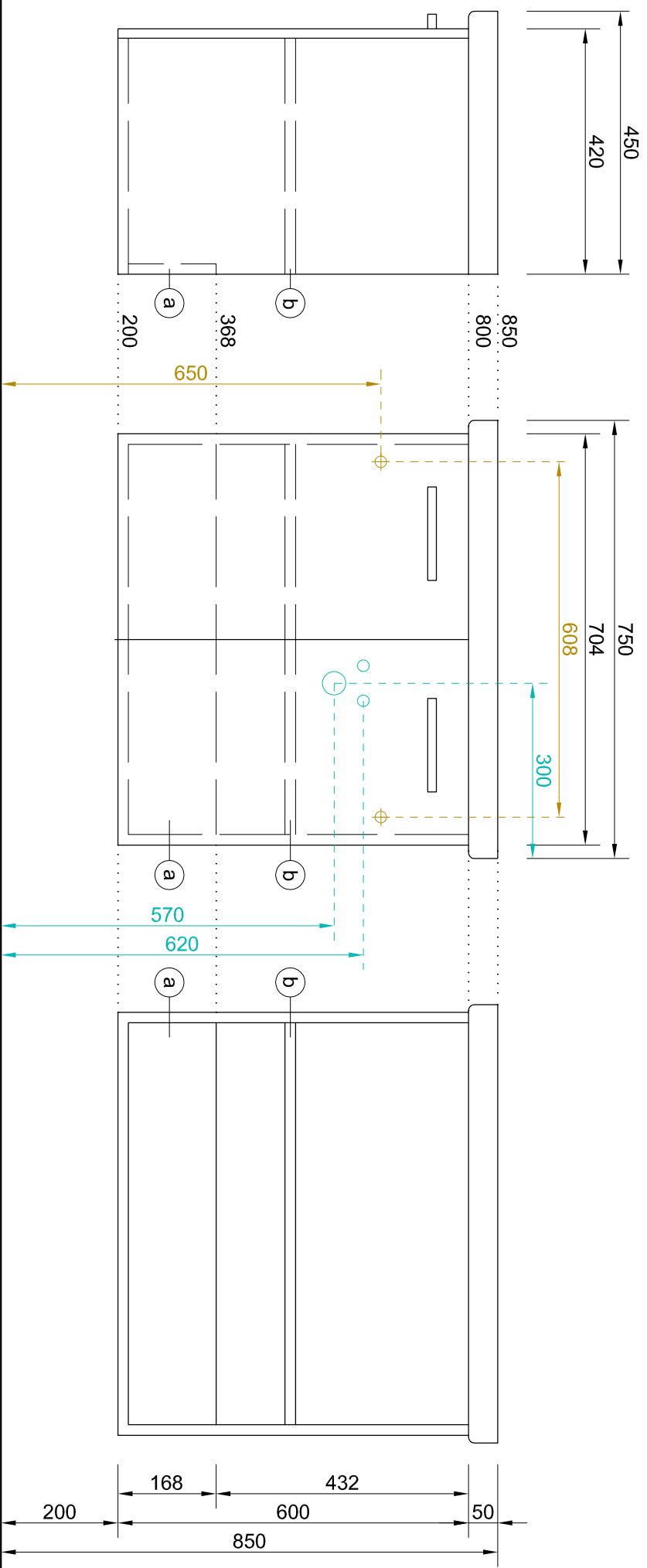
BOČNÍ POHLED
