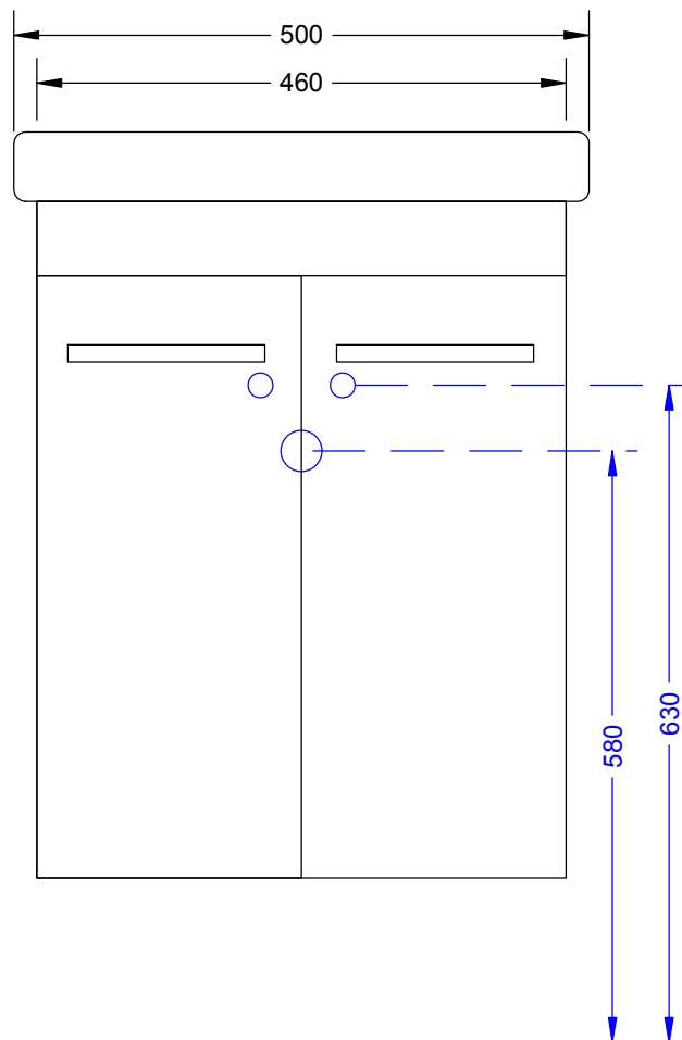
PŘEDNÍ POHLED
