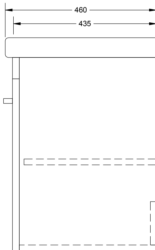
BOČNÍ POHLED
