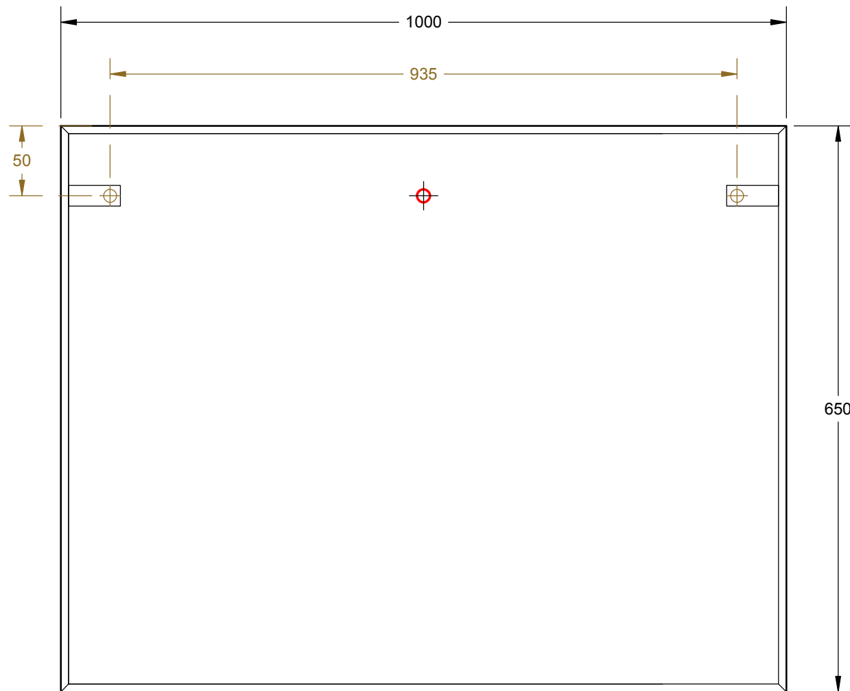
PŘEDNÍ POHLED
