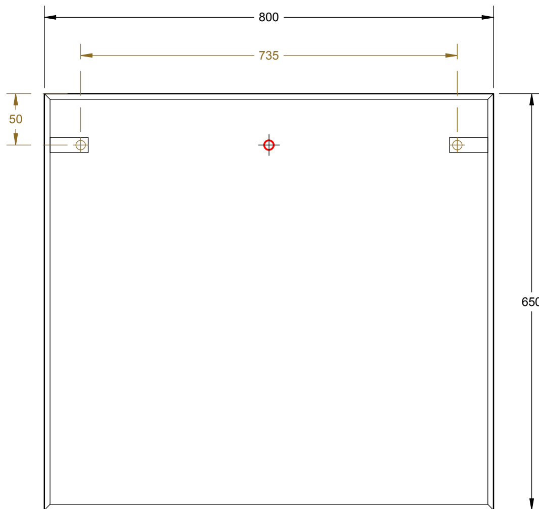
PŘEDNÍ POHLED
