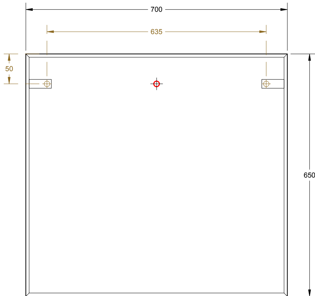
PŘEDNÍ POHLED
